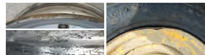
<Jante déformée>
